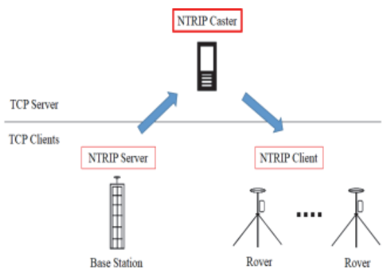
図-4 NTRIP の仕組み
