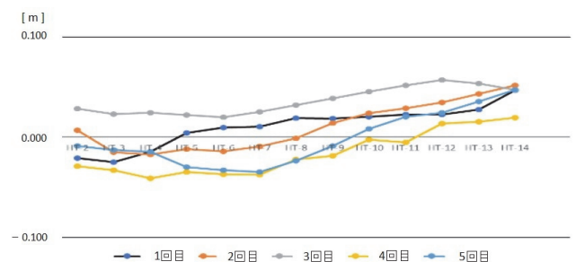
図-6 TS 観測と RTK 観測の Y 座標の較差
