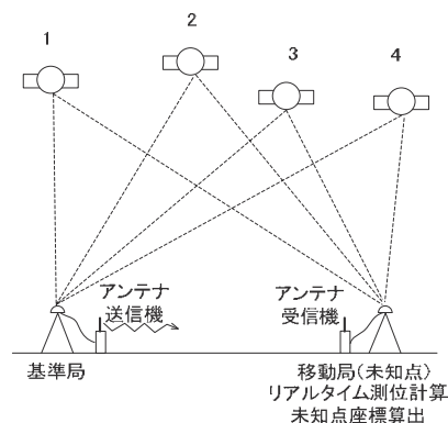
図-2 一般のデイファレンシャル測位
