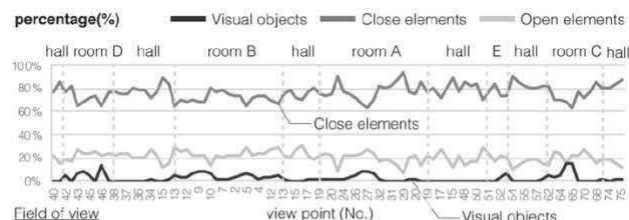
図7 視野範囲における空間構成要素の割合
