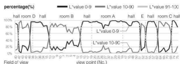
図11 視野範囲における空間明暗要素の割合
