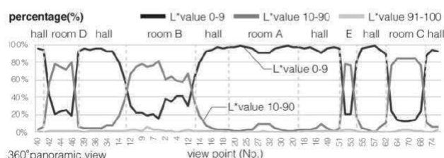
図10 全周範囲における空間明暗要素の割合
