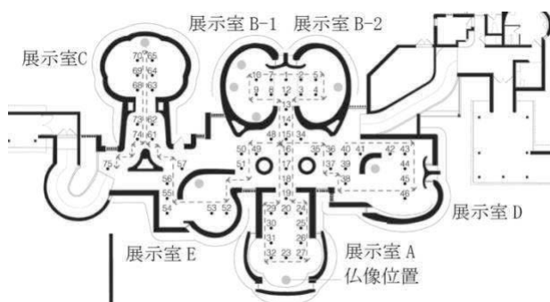
図4 谷村美術館 平面図
