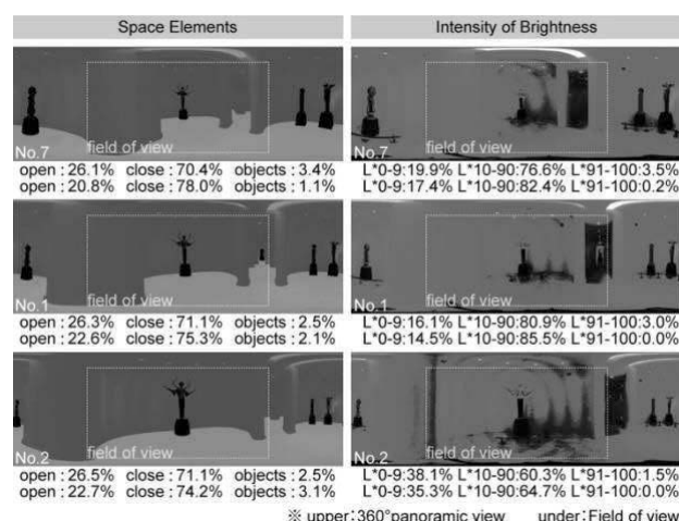
図19 展示室Bの連続写真及び空間要素の割合
