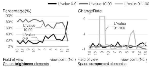
図20 展示室Bの視覚情報の変化のグラフ
