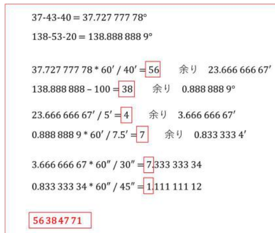
図2 メッシュコードの計算
