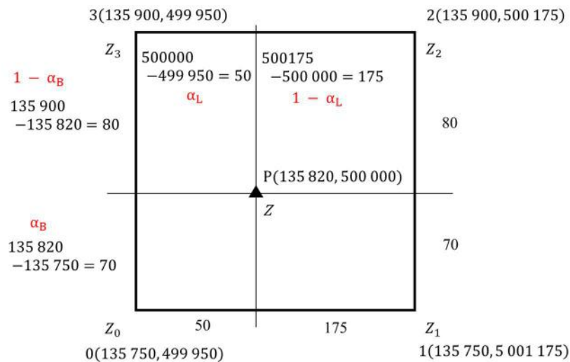
図6 計算例
