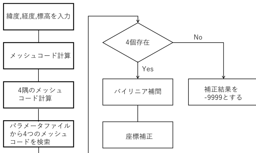
図7 補正計算の流れ
