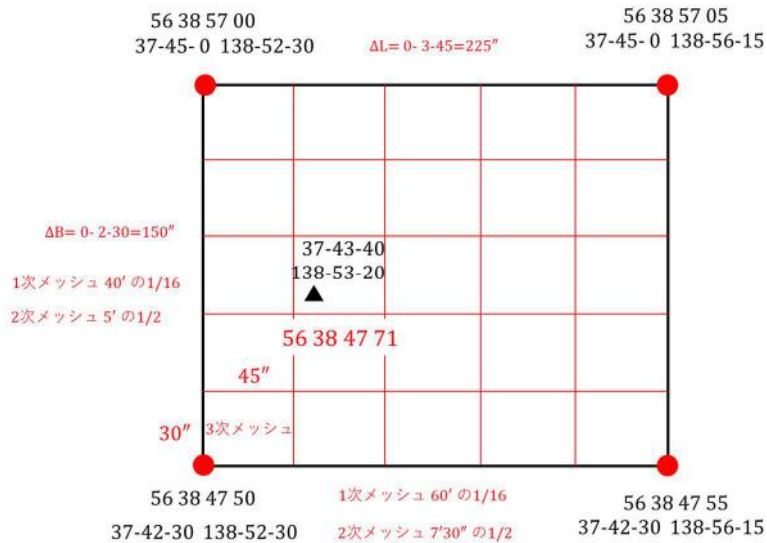
図1 任意点と4隅のメッシュコードの関係
