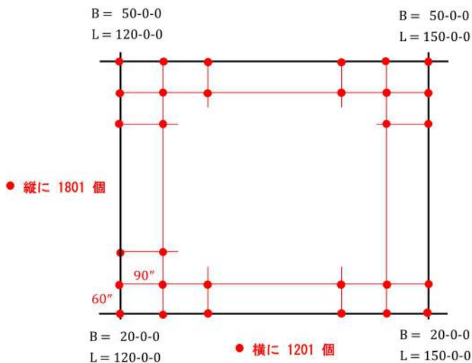
図9 ジオイド・モデルファイルのデータ構造
